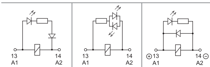
C: 选项3、5、54 LED (交流) C: 选项6、7、74 双排LED (直流非极化) C: 选项8、9、94 LED + 二极管 (直流, 对A1/13针脚为正极性)
