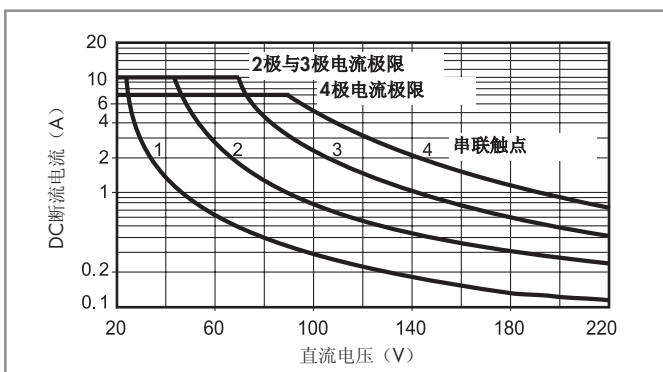
H 55 - 最大DC1断流容量
