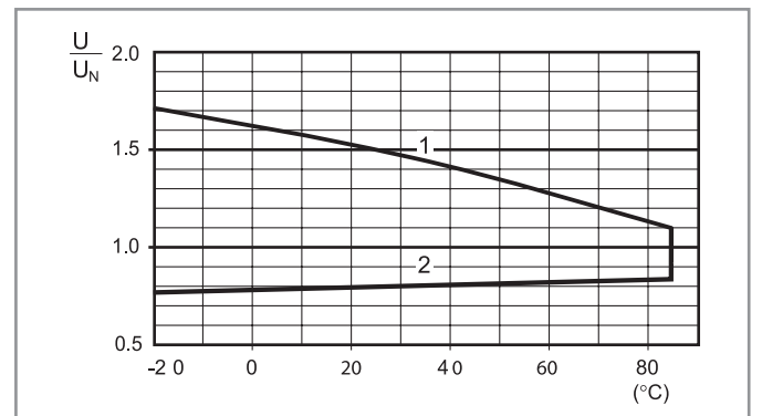
R 55 - 交流线圈工作范围对比环境温度
