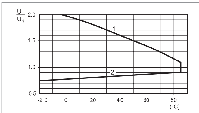
R 55 - 直流线圈工作范围对比环境温度
