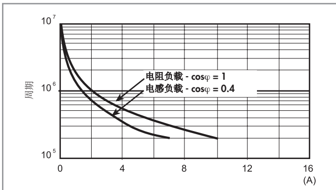
F 55 - 电气寿命 (AC) 对比触点电流 双极继电器和3极继电器
